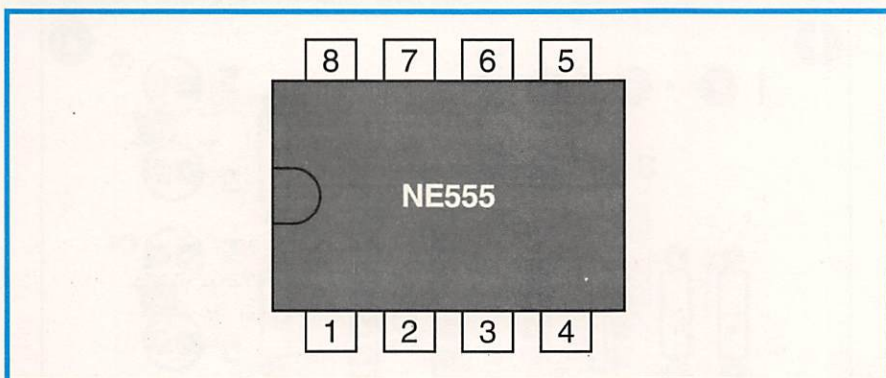
Figure 3b : Brochage du 555 (vue de dessus !).
