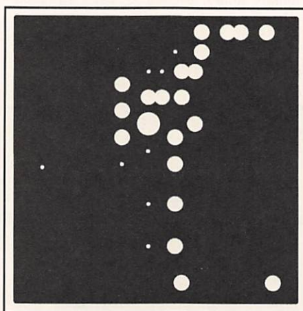
Côté cuivre vu par transparence de la face composants, échelle : 1
