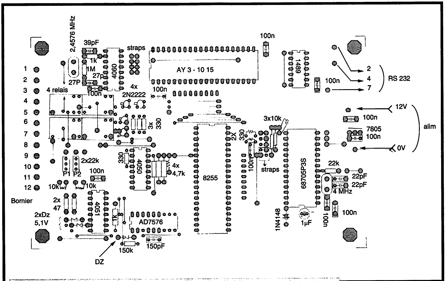
Figure 3. Plan d'implantation des composants.
