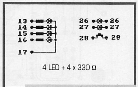
Connexions des LED.
