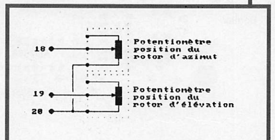
Connexions des potentiomètres.
