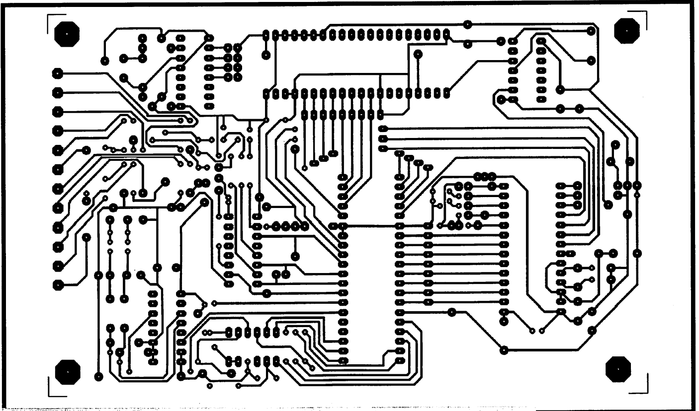
Figure 2. Plan du circuit imprimé échelle 1.
