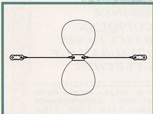
Fig. 3. Lobe de rayonnement du dipôle.
