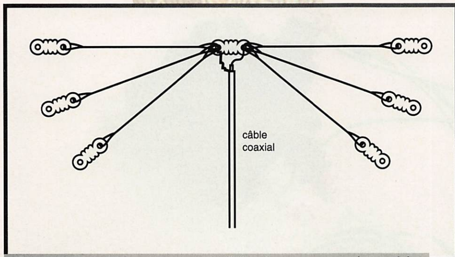
Fig. 1a. Attaque du centre du multi-dipôle directement par le coaxial. Mauvaise adaptation, réglages plus ardues.
