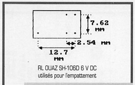
Référence des relais.
