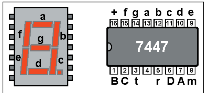
Figure 1 : Brochage d'un afficheur 7 segments et d'un 7447.
